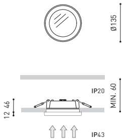
STRAM MINI PRISMATIC
